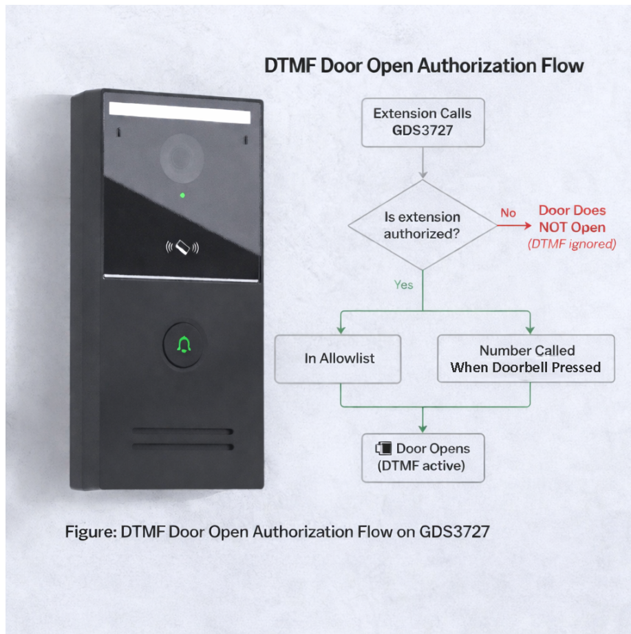
DTMF Door Open Permission
