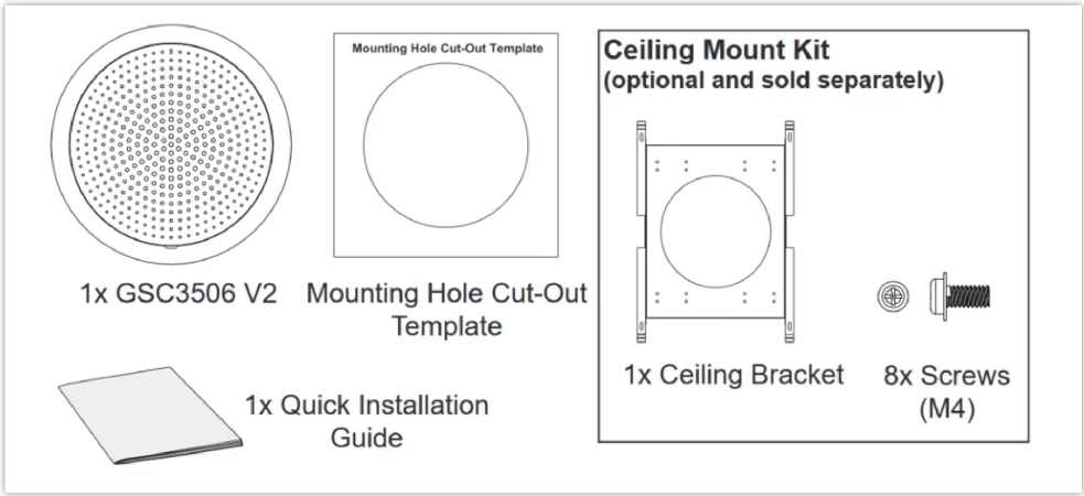
GSC3506 V2 Package Content
